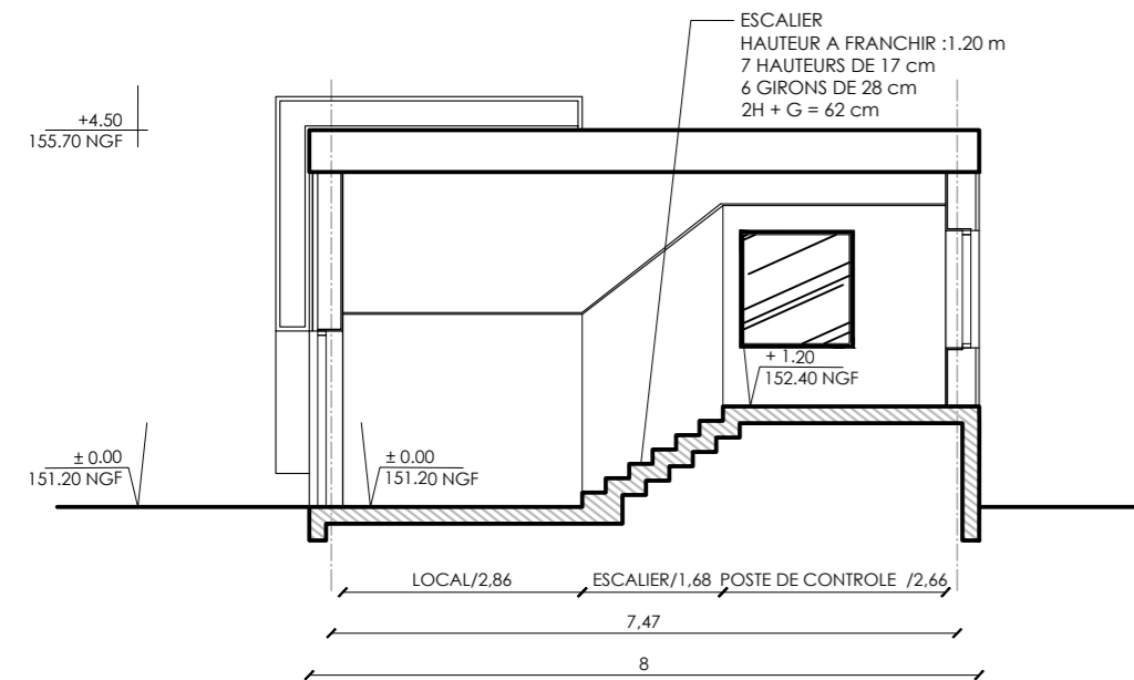
COUPE AA
