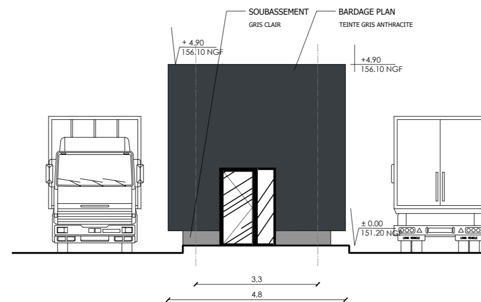
FACADE OUEST
