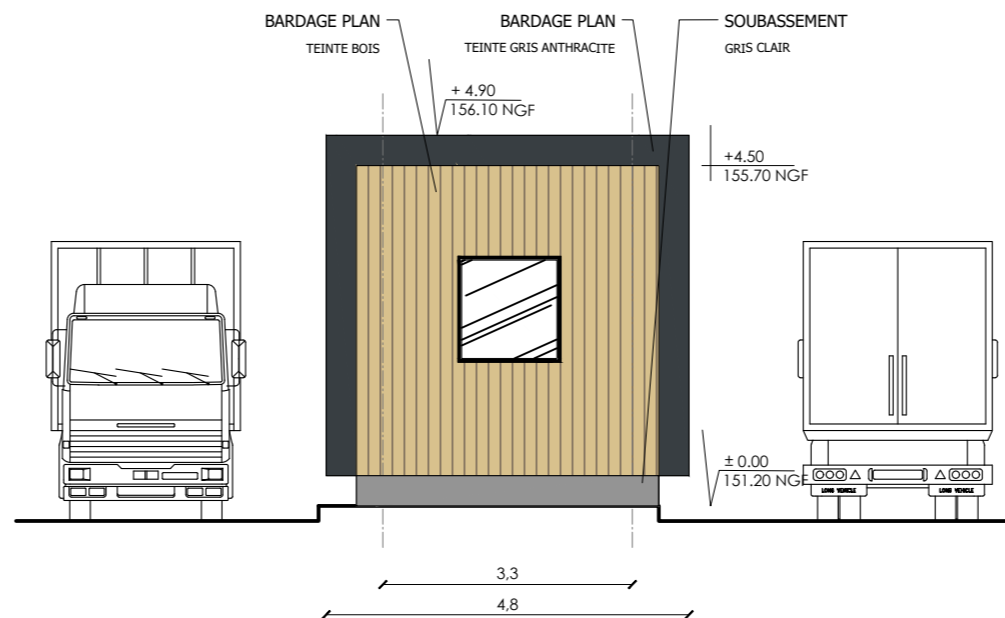
FACADE EST
